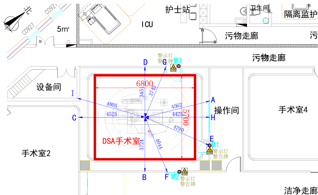
图 11-2 DSA 手术室估算点位示意图
