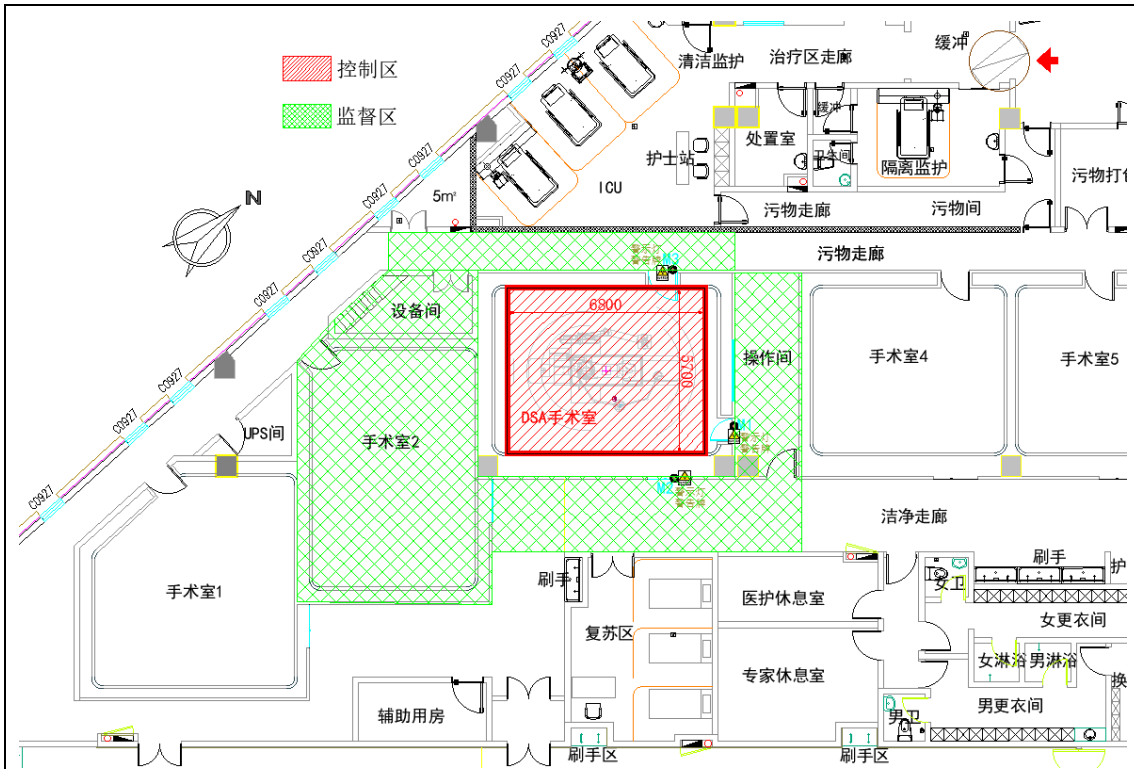
图 10-1 DSA 手术室辐射安全设施布置及分区图
