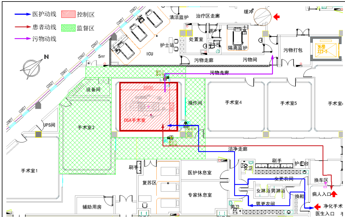
图 11-1 医院 DSA 手术室分区和路由平面布局图
